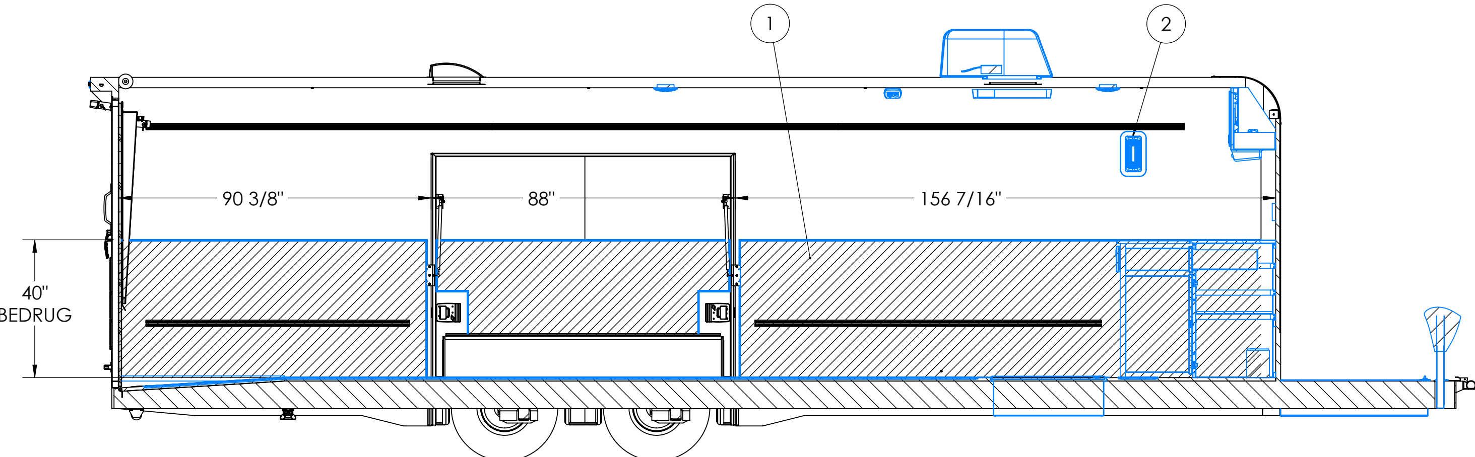
SECTION D-D SCALE 1 : 28
