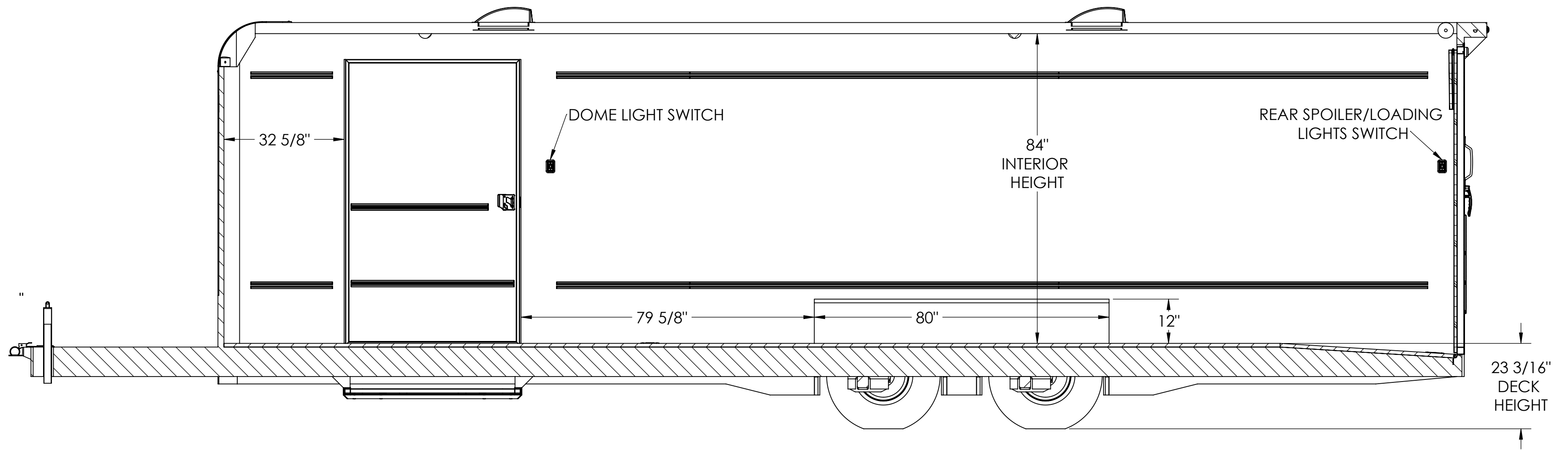
SECTION A-A SCALE 1 : 22
